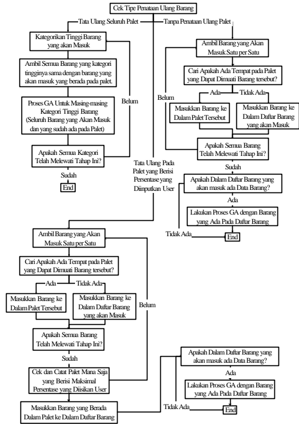
Gambar 11. Algoritma Penambahan Barang Baru
