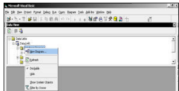
Gambar 5. Pembuatan Diagram
